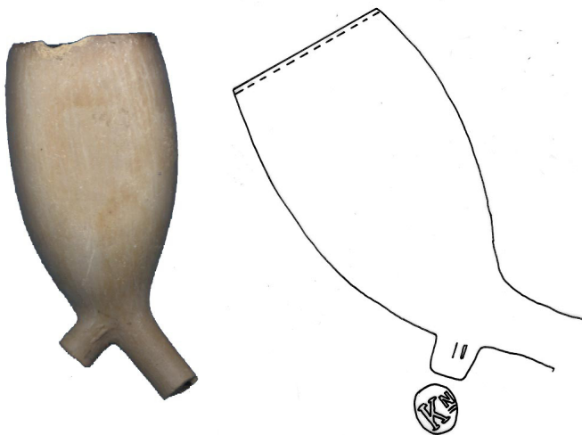
Afb. 9a en 9b. Ovale pijp, hielmerk Kn. Bijmerk zijkant hiel links drie streepjes (gestileerd wapen van Kampen) en hiel rechts een cirkel. Kampen, Frerichs en Steinman, 1829-1830. (Foto en tekening: (c) Jan van Oostveen ( http://kleipijp.home.xs4all.nl ), uit Van Oostveen, 2005, p.30, afb. 25.)
